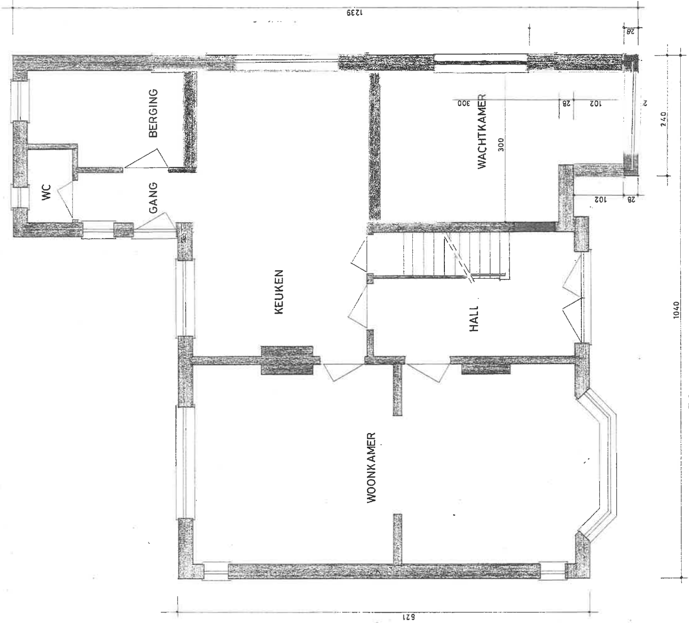
PLAN GELUJKVLOERS 1:50
